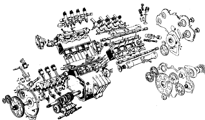
Esploso Motore otto cilindri
